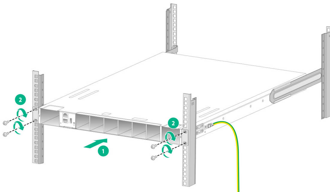
图2-22 安装 S9800-24B8D 和 S9800-32D 以太网交换机到机柜示意图（挂耳安装在靠近电源侧）
