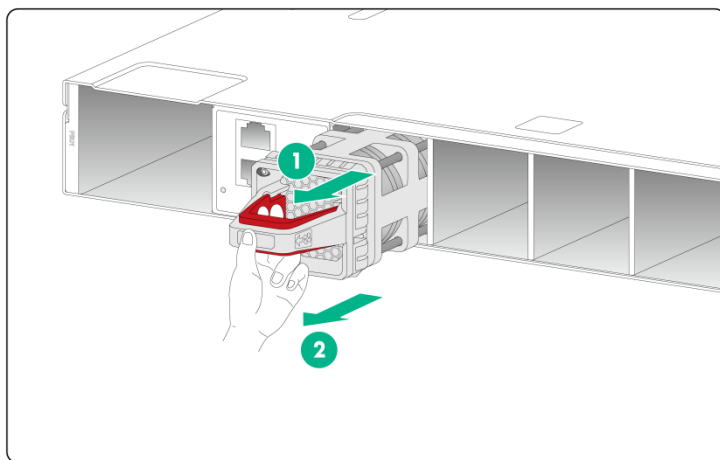
图2-26 FAN-40B-1-H-2-Z 和 FAN-40F-1-D-Z 风扇模块拆卸示意图
