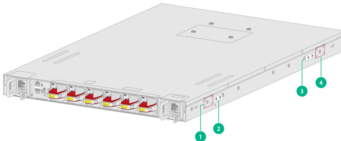
图2-11 挂耳安装位置、接地线缆连接位置
