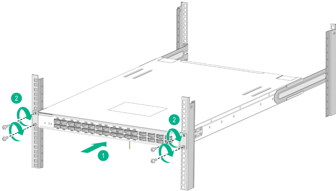
图2-20 安装 S9800-24B8D 以太网交换机到机柜示意图（挂耳安装在靠近端口侧）
