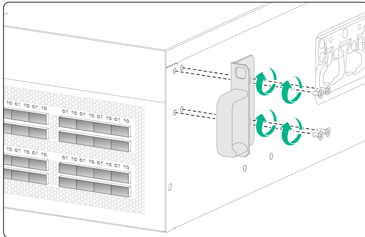
图2-12 安装挂耳到 S9805-64D 机箱
