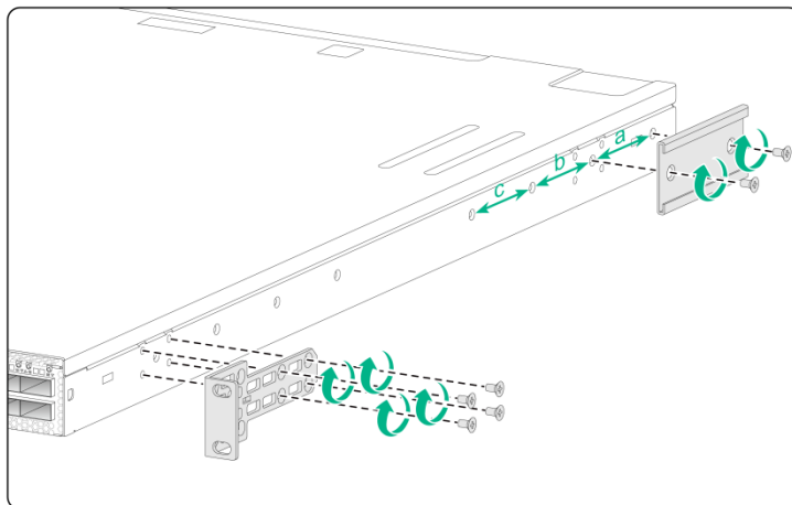
图2-13 安装挂耳和滑道导轨到 S9800-24B8D 和 S9800-32D 机箱（采用端口侧挂耳安装位）
