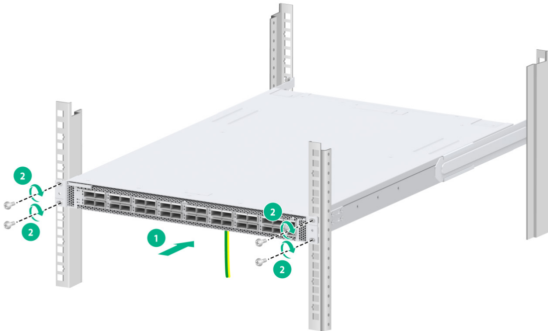
图2-21 安装 S9800-32D 以太网交换机到机柜示意图（挂耳安装在靠近端口侧）
