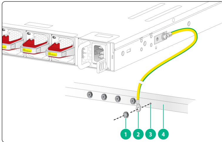
图2-23 连接接地线缆到接地排
