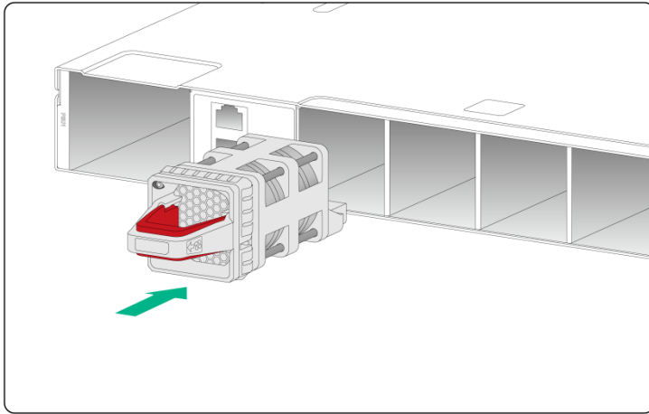
图2-24 FAN-40B-1-H-2-Z 和 FAN-40F-1-D-Z 风扇模块安装示意图
