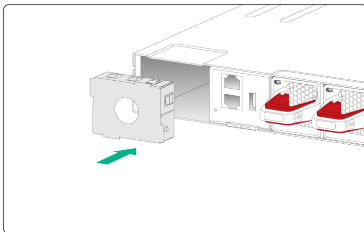
图2-35 电源假面板安装示意图
