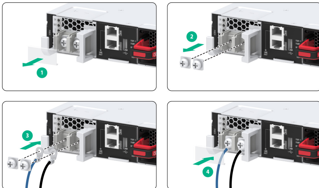
图2-39 PSR2400B-12D-B-Z 直流电源线连接示意图
