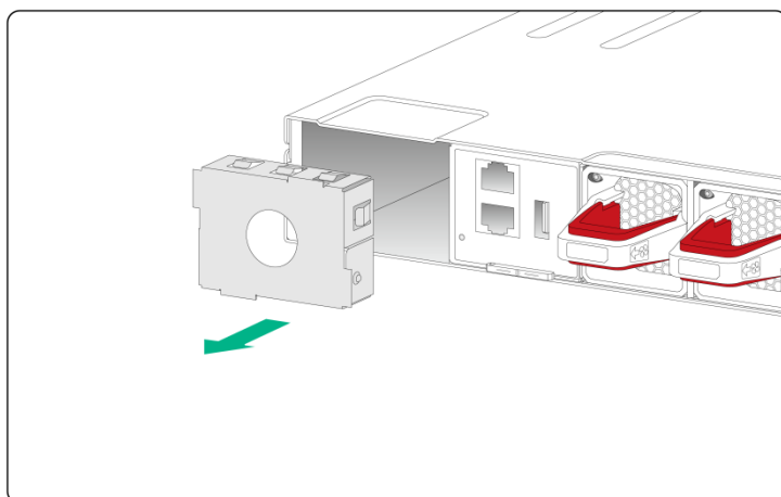
图2-31 电源假面板拆卸示意图
