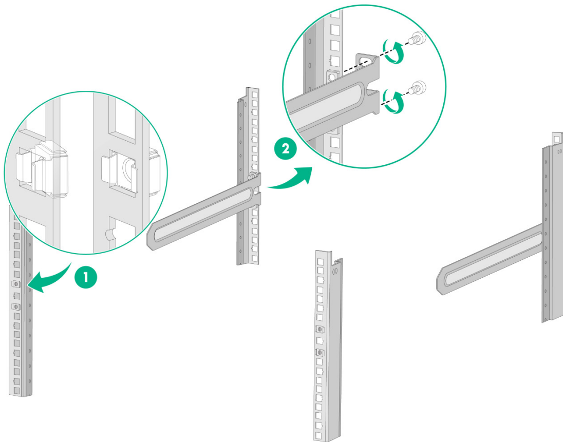
图2-17 1U 滑道安装示意图
