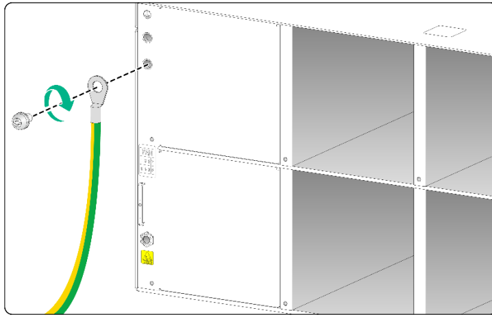
图2-15 安装接地线缆到 S9805-64D 接地点的示意图
