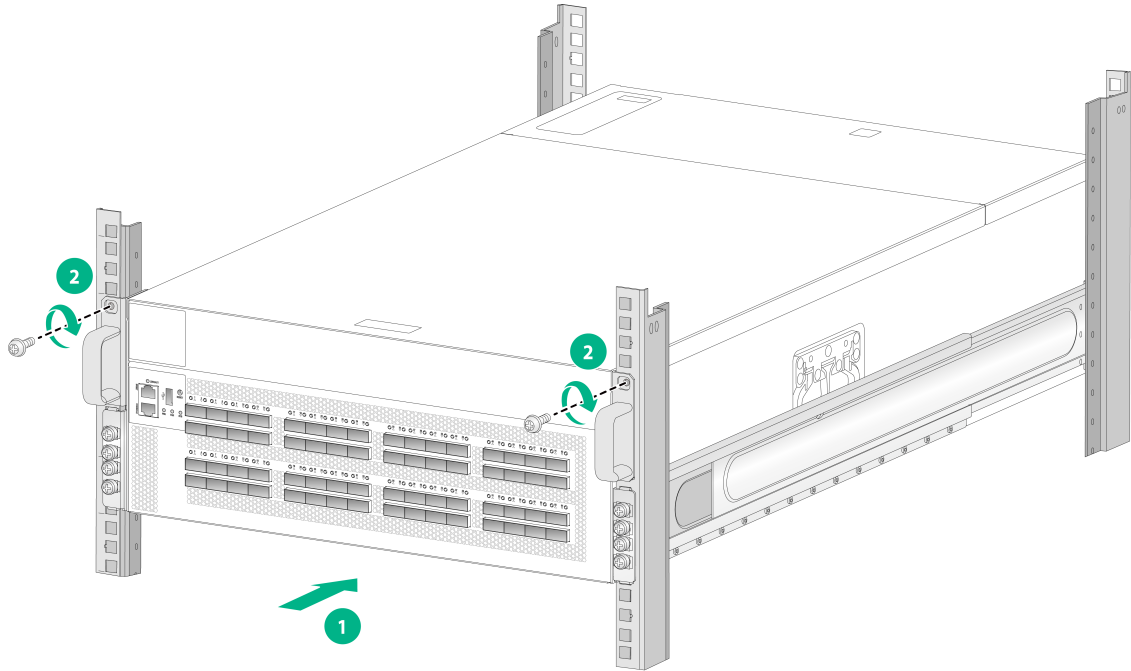
图2-19 安装 S9805-64D 以太网交换机到机柜示意图
