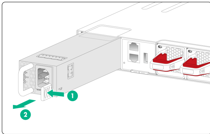
图2-34 拆卸电源模块示意图
