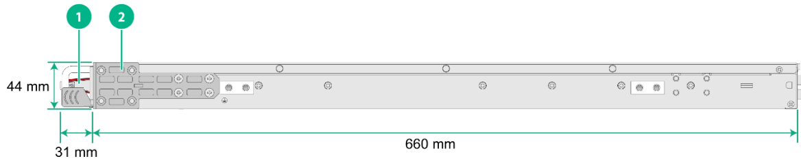
图2-5 挂耳安装在电源侧时尺寸示意图
