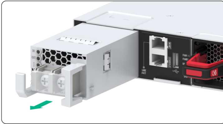
图2-36 拆卸电源模块示意图
