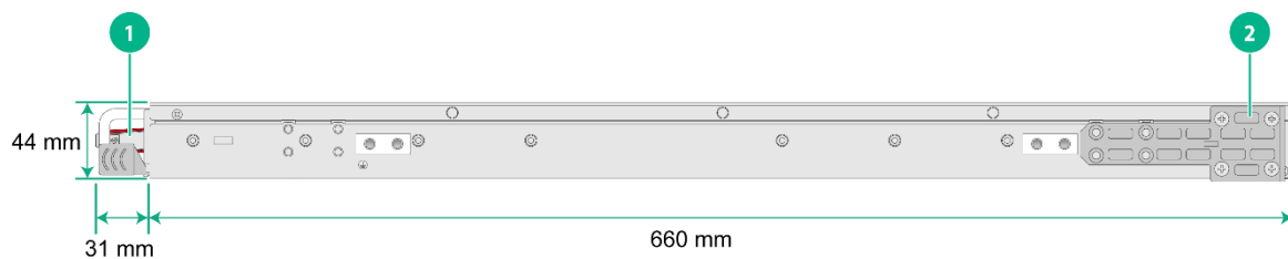
图2-4 挂耳安装在端口侧时尺寸示意图
