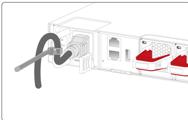
图2-38 PSR1600C-12A-B-Z 交流电源线连接示意图
