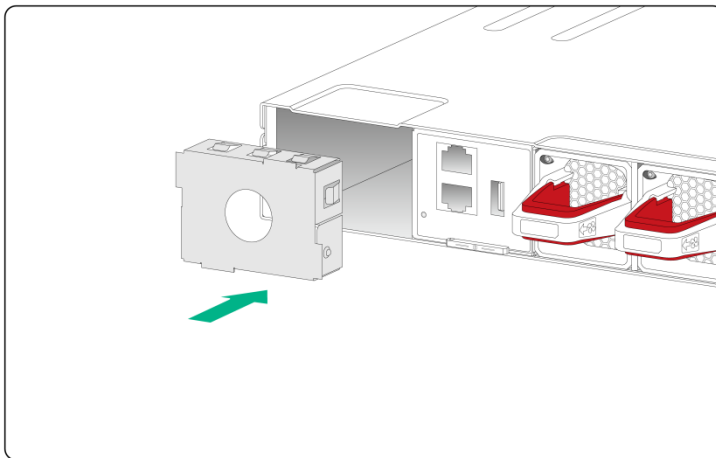
图2-37 电源假面板安装示意图
