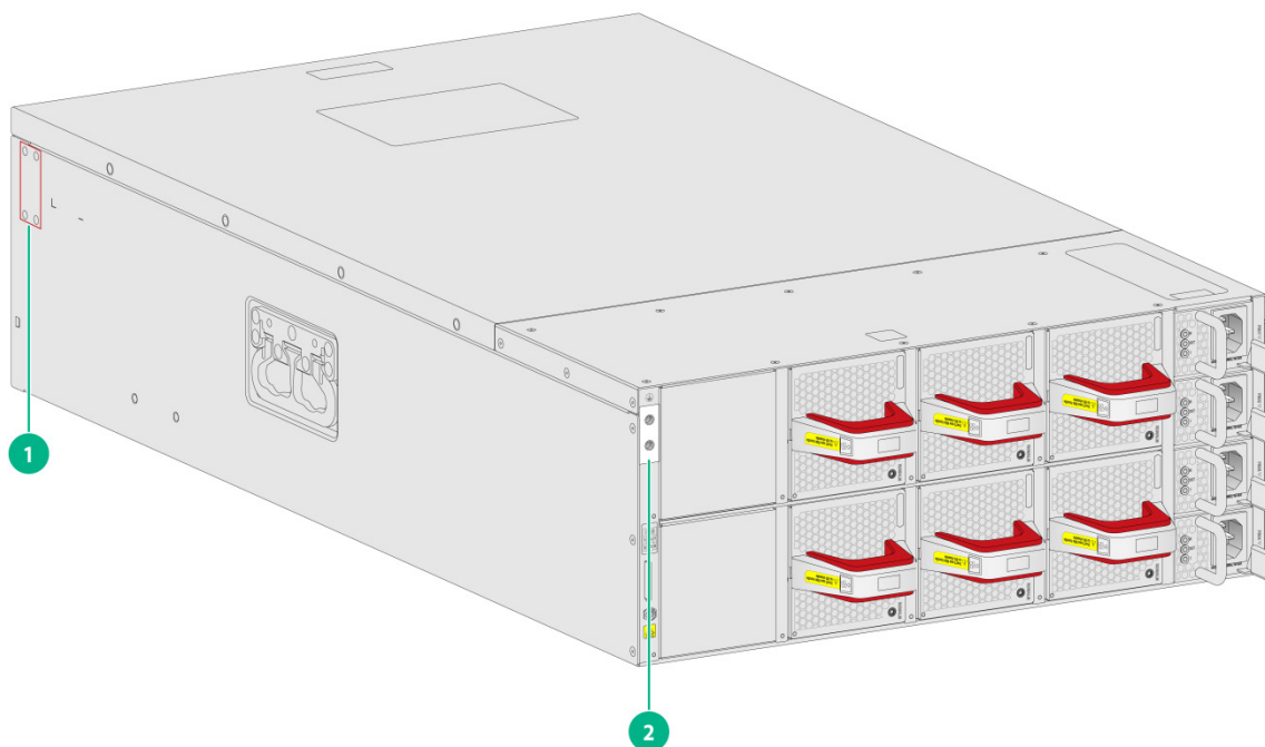
图2-10 S9805-64D 挂耳安装位置、接地线缆连接位置
