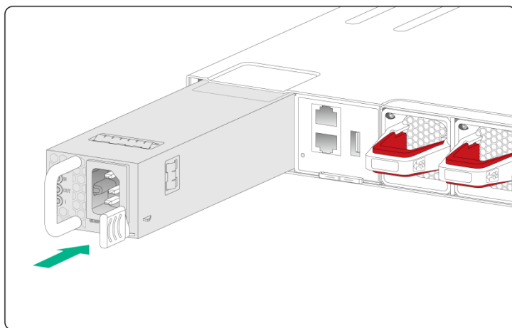
图2-30 电源模块安装示意图
