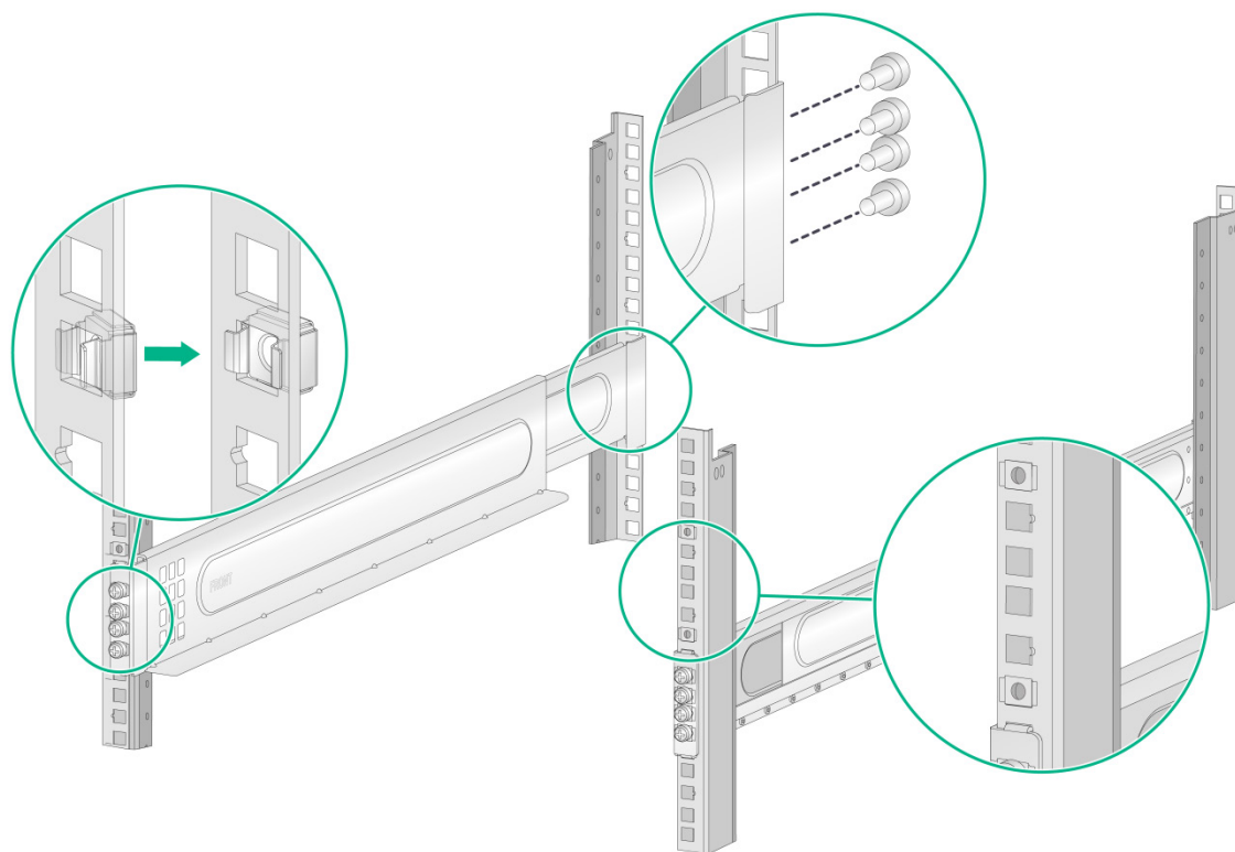
图2-18 可伸缩式滑道安装示意图
