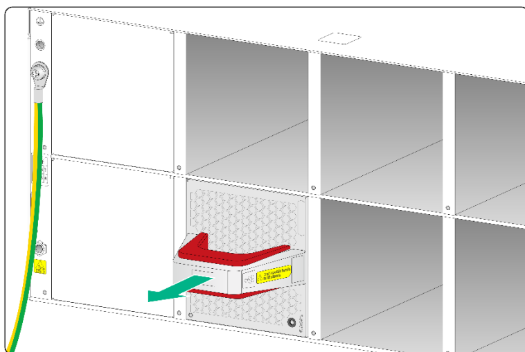
图2-27 FAN-80B-1-B-Z 风扇模块拆卸示意图
