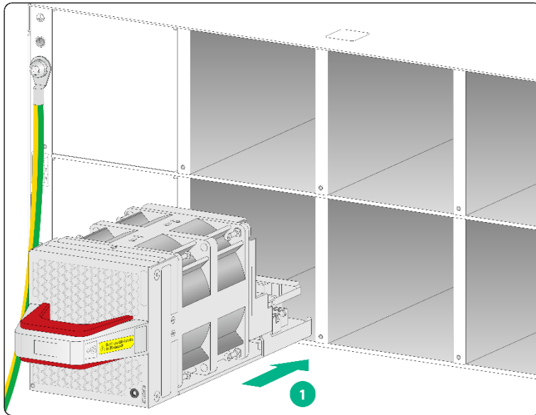
图2-25 FAN-80B-1-B-Z 风扇模块安装示意图
