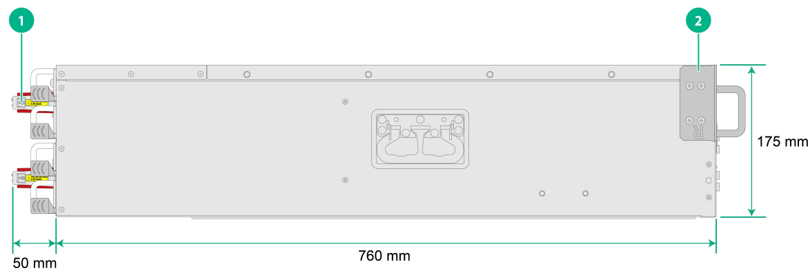
图2-3 S9805-64D 挂耳安装尺寸示意图
