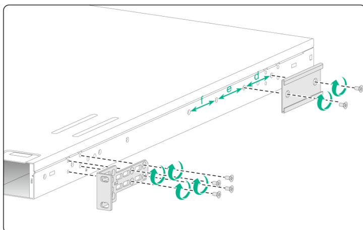
图2-14 安装挂耳和滑道导轨到 S9800-24B8D 和 S9800-32D 机箱（采用电源侧挂耳安装位）
