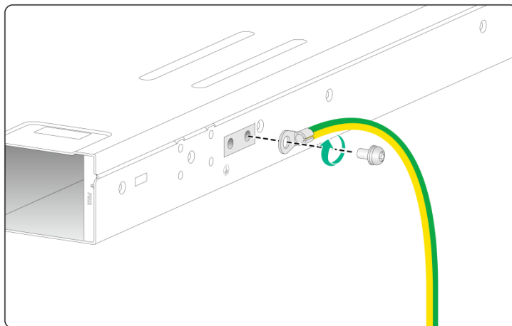
图2-16 安装接地线缆到 S9800-24B8D 和 S9800-32D 主用接地点示意图
